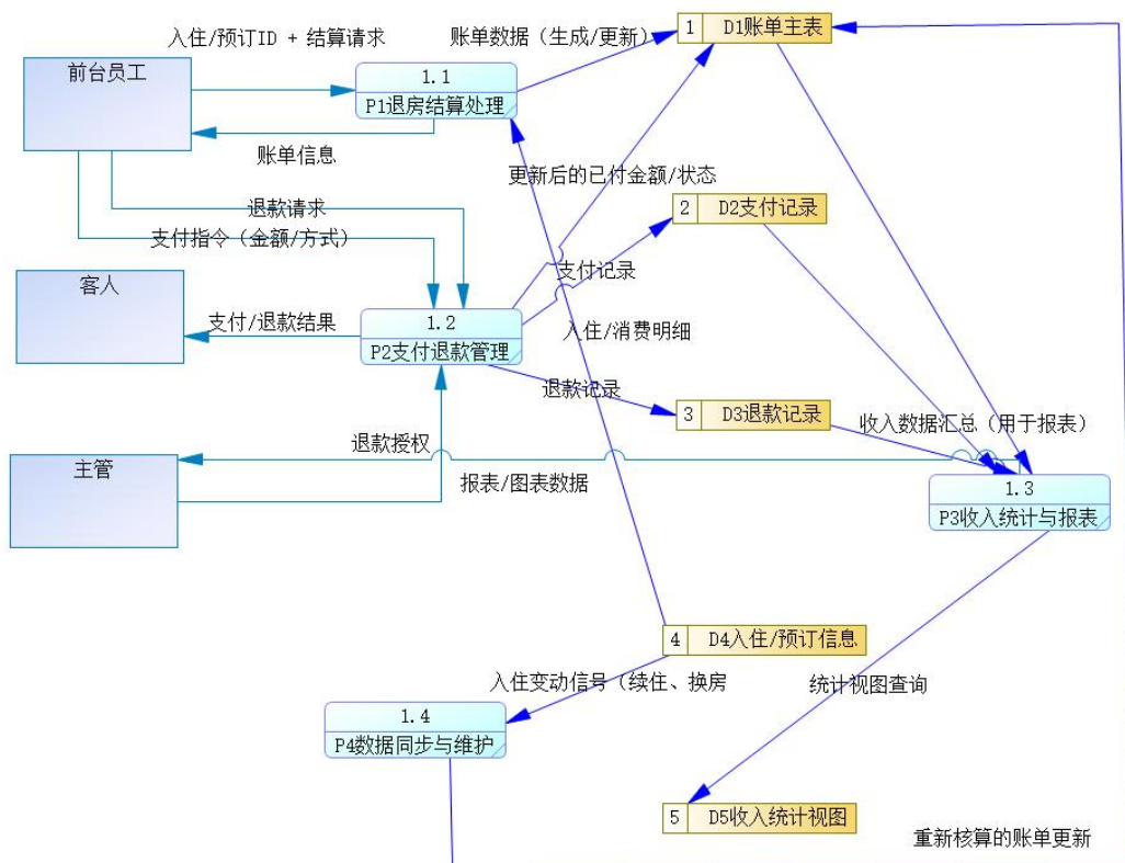
图 5 前台 dfd
