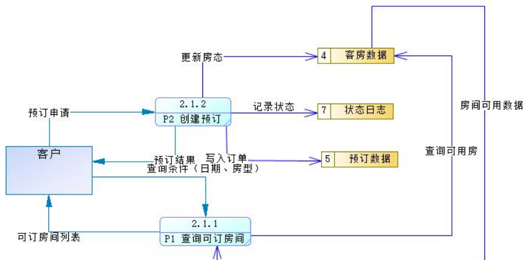
图 3 预定 dfd
